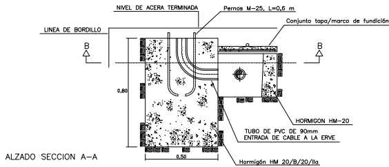
ALZADO SECCION A-A
